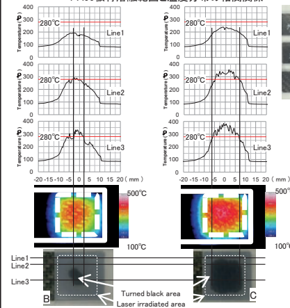
図3. 接合界面の温度条件分析結果
