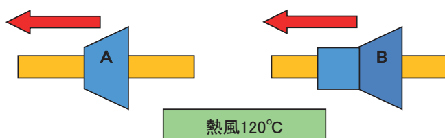
加熱絞りダイスの構造(2種類 A, B)
