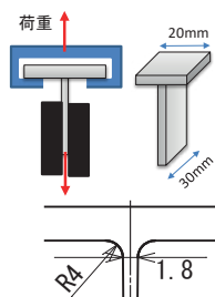
(a) ビレットフロー成形品
