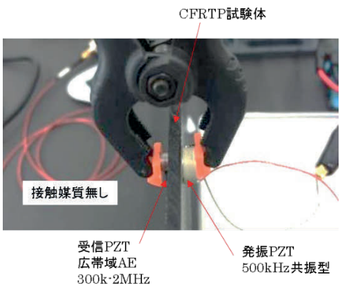
開発した測定プローブ試作品
