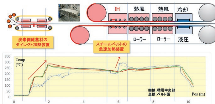
誘導加熱による炭素繊維基材の急速加熱装置を組み込んだ高速成形プロセス
