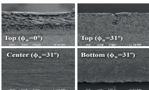
図 加工面性状(SEM)
