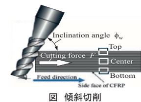
図 傾斜切削
