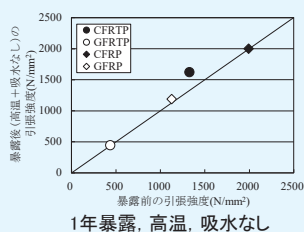
補強筋単体の引張強度
