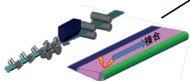
連続成形ブレード
