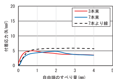
BFRTPIにおける付着応力-すべり量変位曲線 (本数と結束方法による影響)
