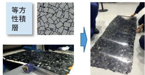
等方性CFテープランダムシート
