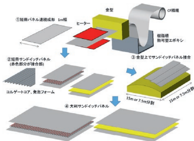
大型平板サンドイッチパネルの連続成形工程
