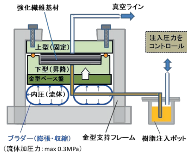
新規・簡易VaRTM装置のイメージ図
