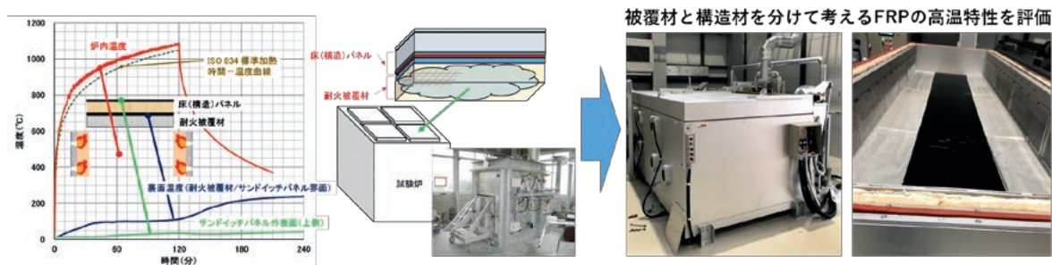
従来の耐火試験と新たに開発した大型高温試験装置
