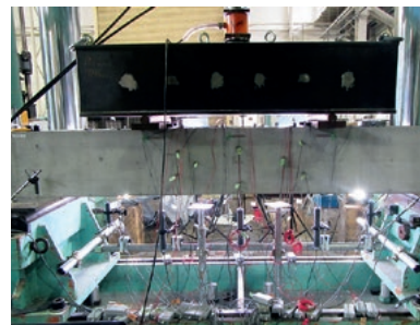
実大規模の載荷試験
