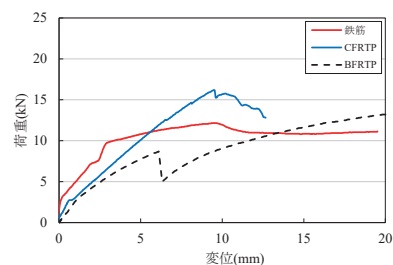
BFRTPIにおける付着応力-すべり量変位曲線 (本数と結束方法による影響)
