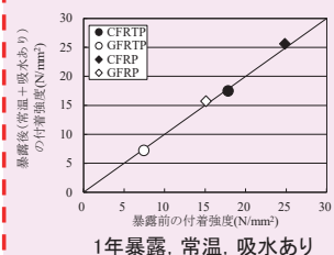
補強筋とコンクリートとの付着強度
