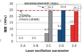
図6. レーザー照射面積(□20mm)で規格化した最大接合強度
