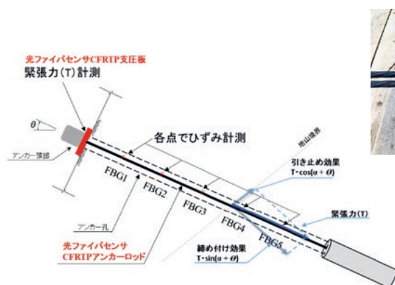
グラウンドアンカーシステム
