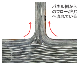
(b) ビレットフロー+パネルフロー成形品
