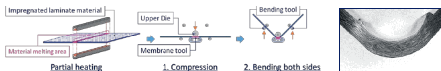
曲げ加工プロセス
