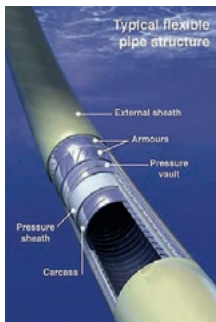
フレキシブルライザー構造図 (Deepflex社ホームページ)
