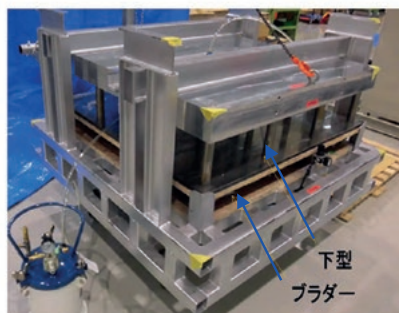
簡易RTM成形試験装置
