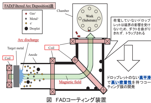
図 FADコーティング装置
