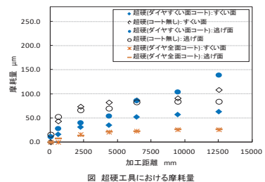
図 超硬工具における摩耗量
