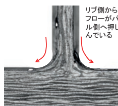
(a) ビレットフロー成形品
