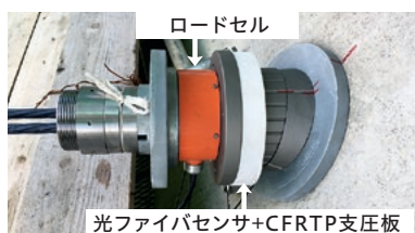
試験施工したCFRTP支圧板
