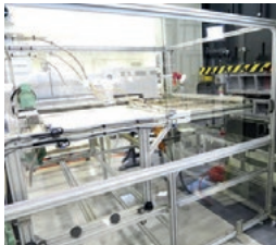
ベルト式加熱搬送装置
